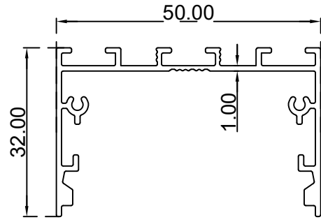
يو انارة (32*50) ملم الرقم التسلسلي للصنف: BLT3618 الوزن (Kg/m): 0.500
