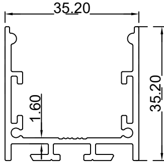
يو انارة (35.2*35.2) ملم الرقم التسلسلي للصنف: BLT3612 الوزن (Kg/m): 0.628
