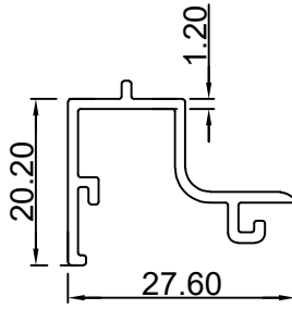
بي عادي 7000 الرقم التسلسلي للصنف: BLT4590 الوزن 0.244: (Kg/m)
