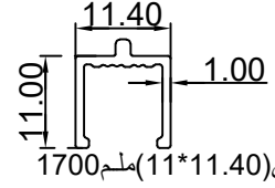
بي (11*11.40) ملم 1700 الرقم التسلسلي للصنف: BLT3799 الوزن 0.103: (Kg/m)
