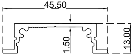
يو انارة (13*45.5) ملم الرقم التسلسلي للصنف: BLT3619 الوزن (Kg/m): 0.337
