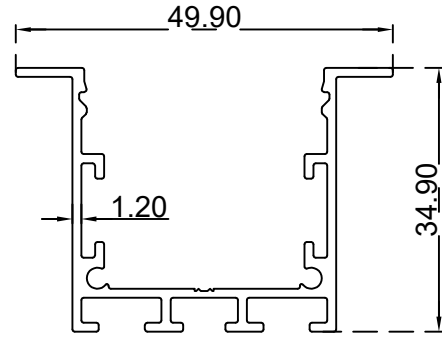
يو انارة (34.9*49.9) ملم الرقم التسلسلي للصنف: BLT3405 الوزن (Kg/m): 0.548
